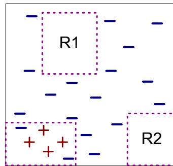
(iv) Step 3
