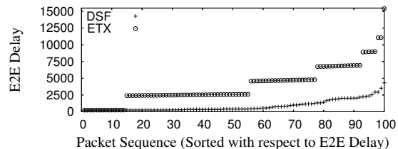
Fig. 16. E2E Data Delivery Delay
